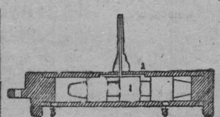
НА СНИМКЕ: перивибратор 1) Ударник, 2) Распределитель, 3) Отверстие для выпуска отработанного пара или воздуха.
