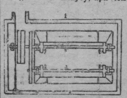
НА СНИМКЕ: Вибратор (вращающаяся площадка) 1) Деревянная площадка, 2) Четырехступенчатые храповики, 3) Валы, на которые насажены храповики.
