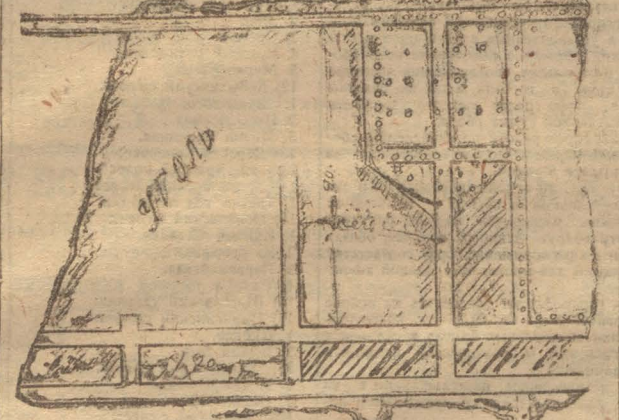
На рисунке — схема выработки Кемеровского пласта по системе, предложенной рабочим Логуновым. (Смотрите его статью в номере от 12 февраля, в технической странице № 6).
