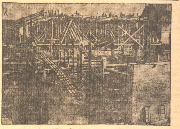
Опалубка бензольного отделения
