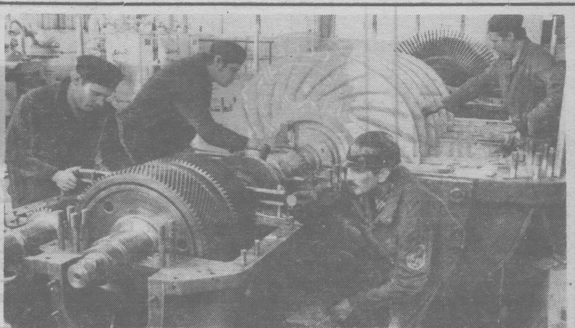
Слесари-наладчики В. Батенев, А. Субботин, Е. Фанюханов, В. Туторов ведут центровку валов трубокомпрессора. Фото П. Костюкова.
