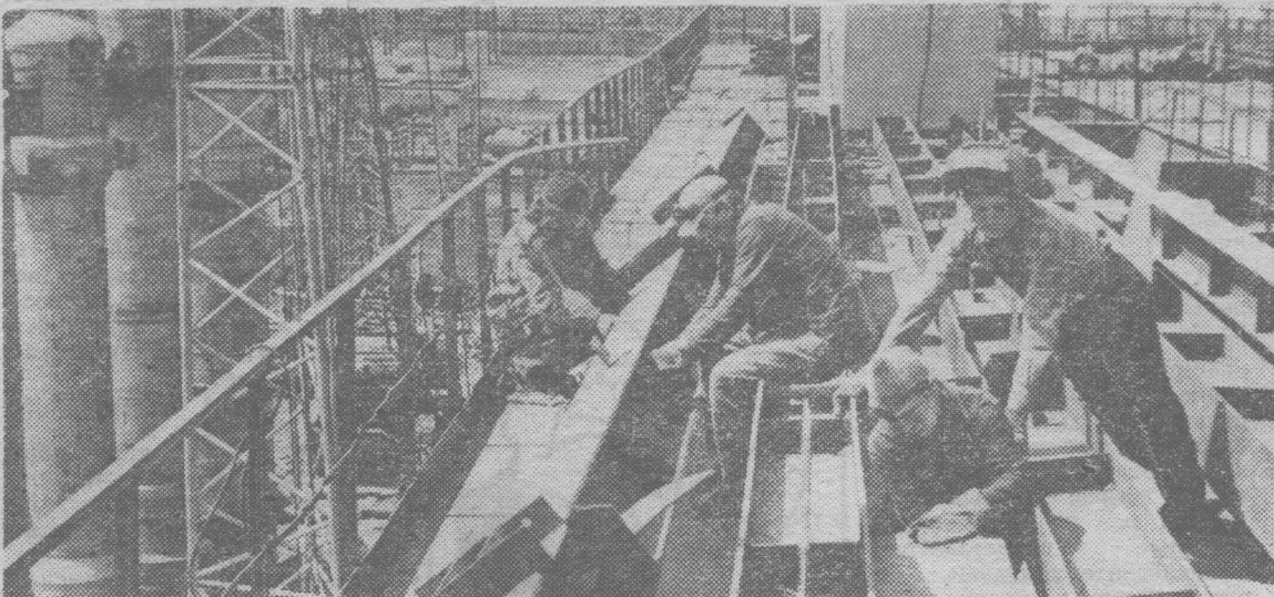
НА СНИМКЕ: идет монтаж металлоконструкций.
