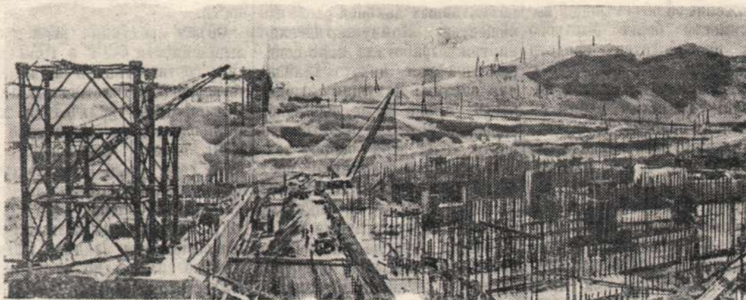
В Таджикистане, близ Ленинабада, на реке Сыр-Дарье строится крупнейшая в Средней Азии Кайраккумская гидроэлектростанция. На снимке: общий вид строительства водосливной плотины и здания Кайраккумской гидроэлектростанции.
