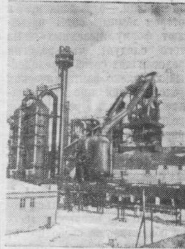
Чкаловская область. На Ор- ско-Халиловском металлурги- ческом комбинате недавно была задута доменная печь по вып- лавке высококачественного при- роднолегированного чугуна. На снимке: новая доменная печь.
