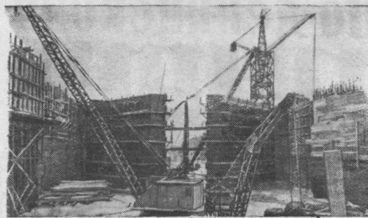
На всех участках строительства Горьковской ГЭС ширится соревнование за досрочную сдачу гидротехнических сооружений в эксплуатацию. На площадке наступает предпусковой период. Полным ходом идет подготовка к перекрытию русла Волги.
