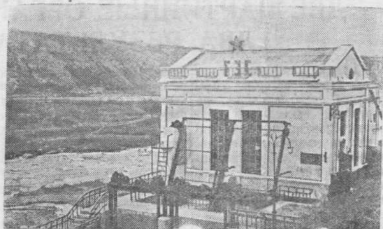
В Николаевской области на реке Южный Буг сооружена Константиновская межколхозная гидроэлектростанция мощностью 800 киловатт. В строительстве ГЭС принимали участие колхозы Арбузинского и Доманевского районов. Первые 14 колхозов уже получили электрический ток для освещения домов и для нужд колхозного производства.
