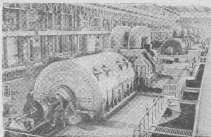
Сталинская область. На строительстве Славянской ГРЭС заканчивается монтаж турбины и двух котлов. Скоро мощность электростанции значительно возрастет. На снимке: турбинный зал Славянской ГРЭС.
