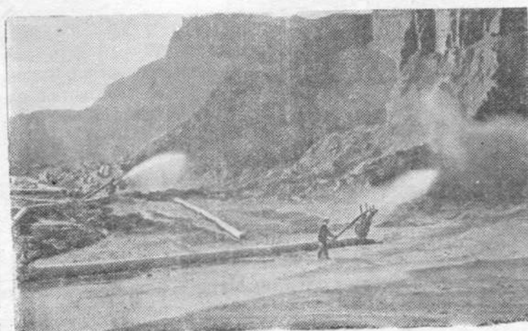
Челябинская область. На Батуринском угольном разрезе № 3—4 треста «Коркинуголь» наряду с экскаваторными работами широко применяется гидромеханизация на вскрыше и добыче угля. Этот метод комплексной механизации позволяет разрабатывать и транспортировать породу и уголь, обогащать его и убирать отходы в отвал. Гидромеханизаторы Батуринского разреза систематически перевыполняют план.
