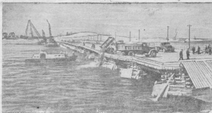
Горьковская область. Для перекрытия русла Волги на строительстве Горьковской гидроэлектростанции сооружен понтонный мост шириной в 20 метров и длиной в 300 метров, с которого автомосвалы сбрасывают камень.
