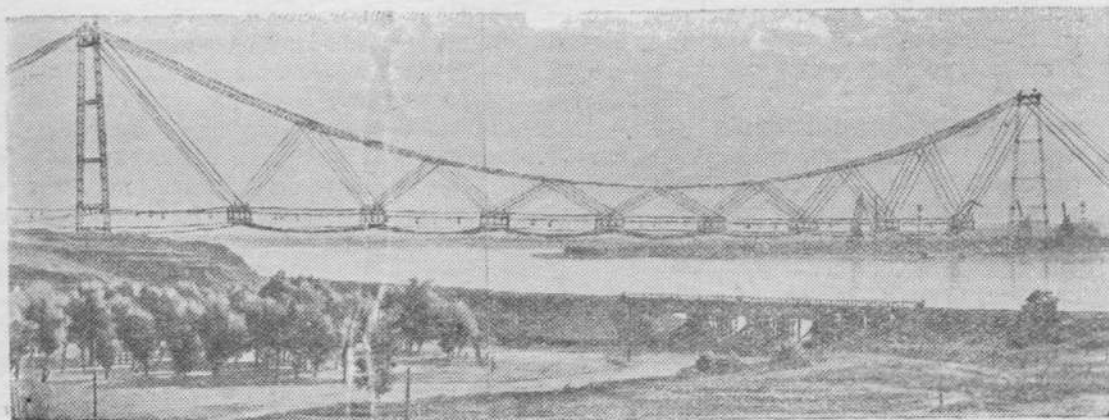
Сталинградская область. Для обеспечения районов строительства Сталинградской гидроэлектростанции щебнем и песком над Волгой сооружена подвесная канатная дорога.
