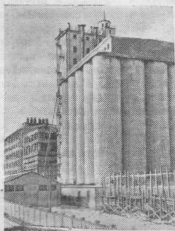
Молотов. На берегу Камы сооружается крупнейший на Урале мелькомбинат, который начнет работать в текущем году. Разгрузка зерна из барж будет производиться с помощью пневматической установки. На снимке: строительство мелькомбината.
