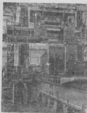
На Горьковском заводе фрезерных станков изготовлен универсальный продольно-фрезерный станок. Вес его — 330 тонн. По высоте он равен двухэтажному дому. Станок оснащен несколькими мощными моторами и будет обрабатывать детали весом до 120 тонн.
