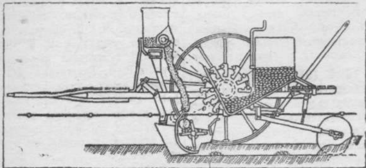
Рис. 1. Схема машины «СКГ-4» для квадратно-гнездовой посадки картофеля.
