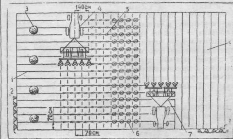
Рис. 3. Схема квадратно-гнездовой посадки картофеля под культиваторы-окушники «КОН-28» и «КУТС-28Б».
