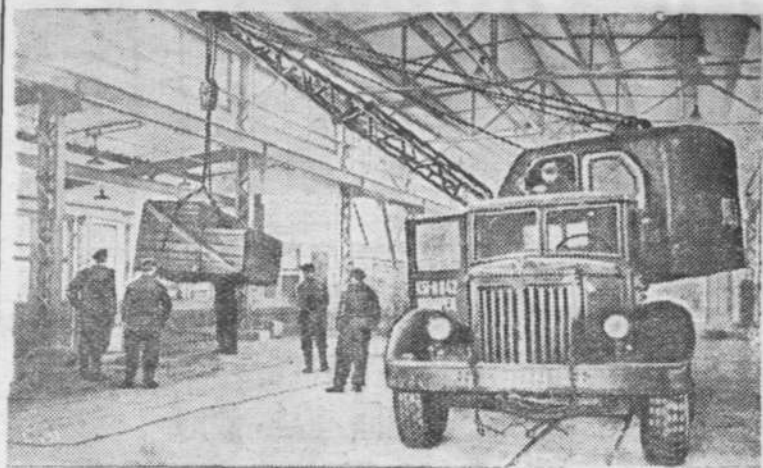
Ленинградская область. Непрерывно увеличивается машинный парк Осьминской МТС.
