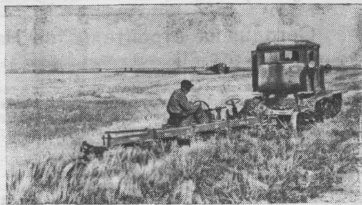
Белорусская ССР. В колхозе имени Гастелло выделен опытный участок, который обрабатывается по методу Т. С. Мальцева. Для этой цели механизаторы Минской МТС сняли у пятикорпусного плуга «П5-35» отвалы и предплужники, отрегулировали плуг для вспашки на глубину 40—45 сантиметров.
