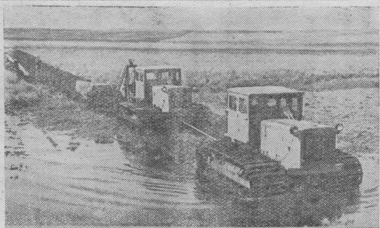
На Челябинском тракторном заводе недавно создан новый мощный болотоходный трактор «С-100Б». Он обладает проходимостью в два раза большей, чем трактор «С-80». На нём установлен дизельный двигатель в сто лошадиных сил.
