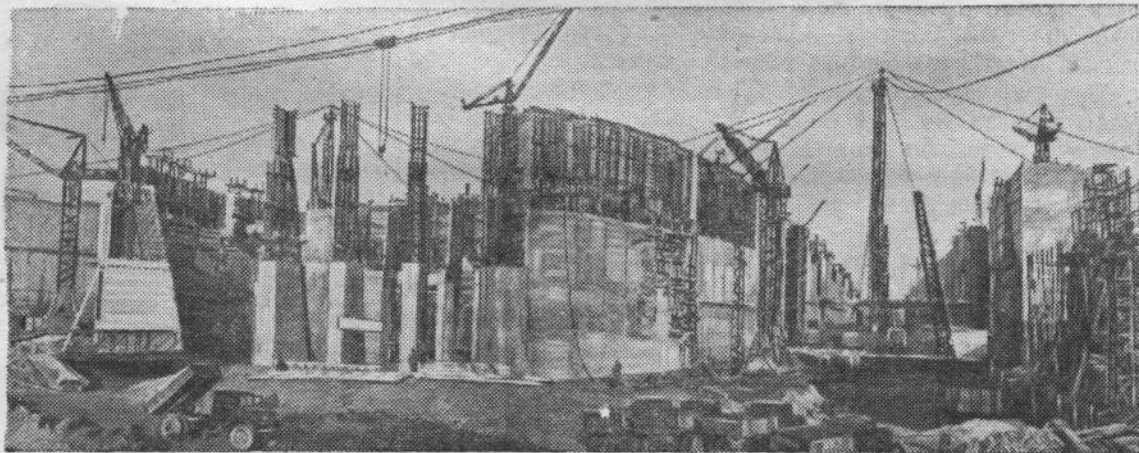
Куйбышевгидрострой. Первый пусковой объект Куйбышевского гидроузла — нижние судоходные шлюзы — вступает в строй весной этого года. День и ночь на громадной территории шлюзов кипит работа. Ведется укладка бетона на самых верхних ярусах, монтируется арматура, устанавливаются основные механизмы управления.
