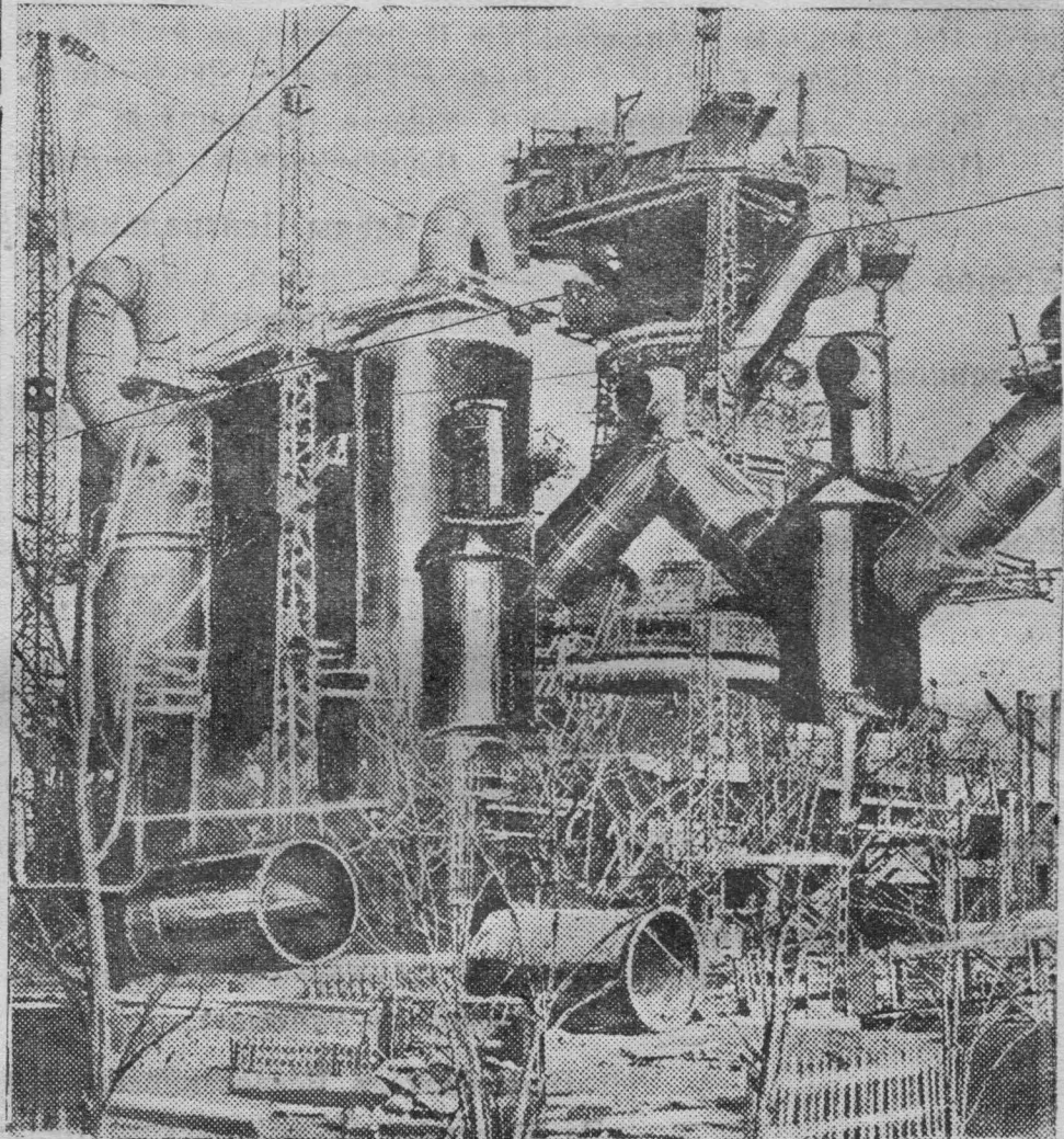
Советская металлургия обогатится в этом году тремя самыми крупными в Европе домнами, которые строятся в Запорожье, Кривом Роге и Мариуполе („Азовсталь“). Объем каждой из новых доменных печей—1300 куб. метров. На снимке: монтаж новой домны на Криворожском металлургическом заводе.
