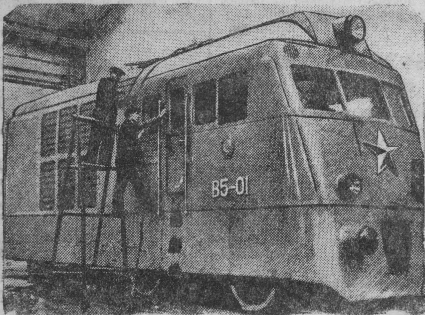
Коломенский машиностроительный завод имени В. В. Куйбышева заканчивает монтаж и сборку основных узлов опытного паровоза высокого давления обтекаемой формы. Этот паровоз даст большую экономию топлива. На снимке: паровоз высокого давления „В5—01“. Слесари сборщики гг. Н. И. Голубков и Н. Г. Федотов заканчивают отделку паровоза.
