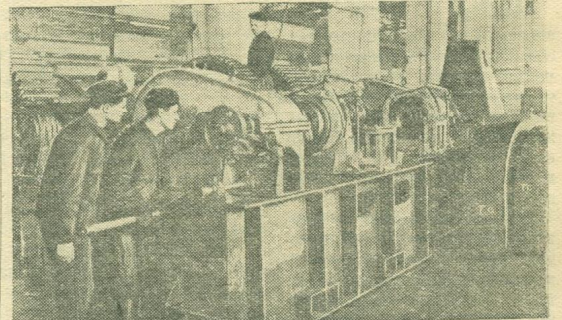
Московская область. Новокраматорские машиностроители закончили сборку механизма шлюзовых ворот Куйбышевской гидроэлектростанции, сократив срок его изготовления на 300 часов против нормы. При выполнении этого почетного заказа больших успехов добились сборщики т. Солнышкин Макаров, Рузин. В течение января-февраля завод изготовил 4 комплекта таких механизмов.
