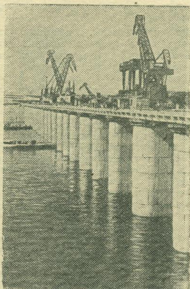
Каховский гидроузел. Водосливная плотина. Фотохроника ТАСС.
