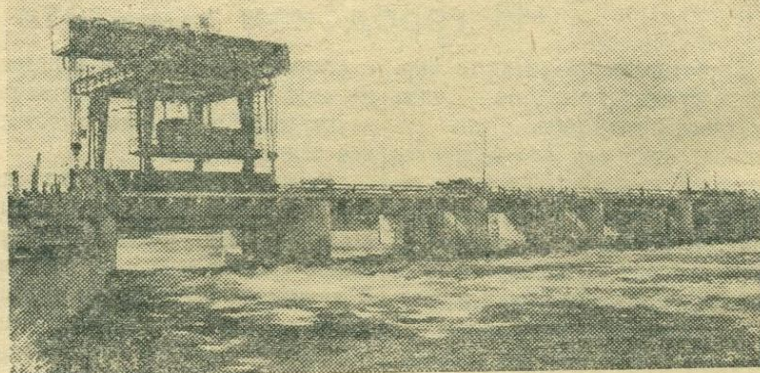
На снимке: водосливная плотина Нарвской ГЭС.
