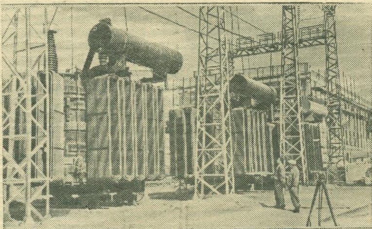
Московская область. В районе Ногинска заканчивается строительство подстанции, предназначенной для приема электроэнергии с Куйбышевской гидроэлектростанции. Первоначальное напряжение в 400.000 вольт здесь будет понижаться до 220.000 и 110.000 вольт. Подстанция полностью оснащена отечественным оборудованием.
