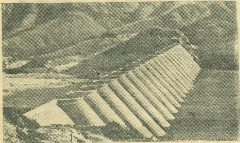
Китайская Народная Республика. Фощэлинское водохранилище на реке Бихэ (провинция Аньхуэй). Его емкость—470 миллионов кубических метров воды.
