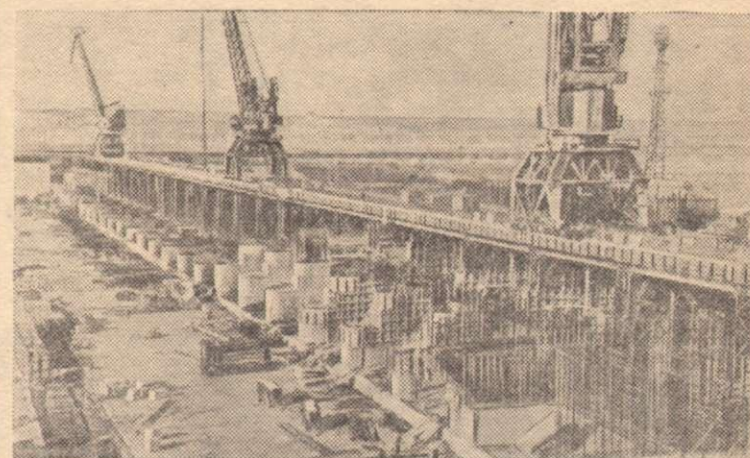
Строители Каховского гидроузла борются за досрочный пуск гидроэлектростанции в 1955 году. Полным ходом идёт сооружение судоходного шлюза, водосливной плотины и здания гидроэлектростанции. Уже установлены статоры четырёх турбин. С опережением графика ведутся монтажные и бетонные работы. На снимке: на участке строительства водосливной плотины. Фотохроника ТАСС.
