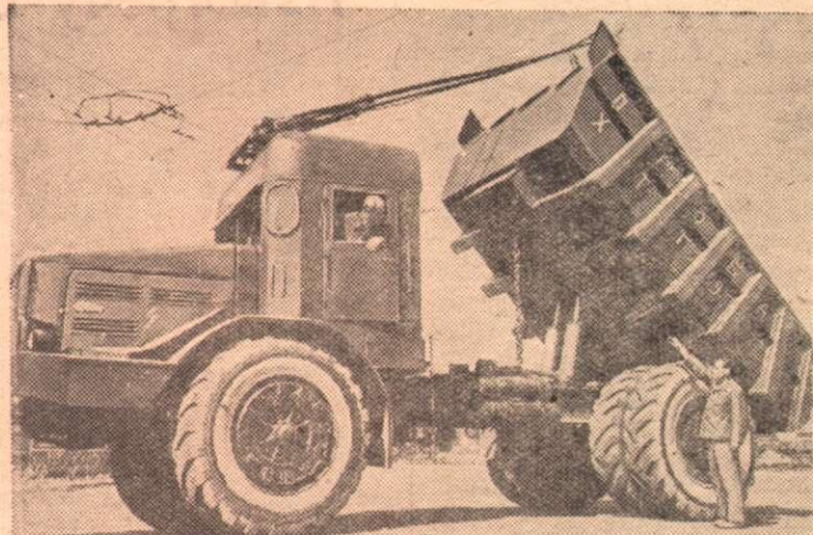
Учёные института горного дела имени М. М. Федорова Академии наук УССР в содружестве с работниками треста «Союзруд» и коллективом Харьковского трамвайно-троллейбусного управления создали на базе автомобиля «МАЗ-525» новый вид грузового транспорта — 25-тонный троллейвоз-самосвал. Эта машина предназначена для работы на предприятиях горной промышленности — в карьерах и рудниках.
