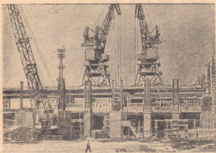
Новая Каховка. На строительстве Каховского гидроузла монтируется первая турбина гидроэлектростанции.
