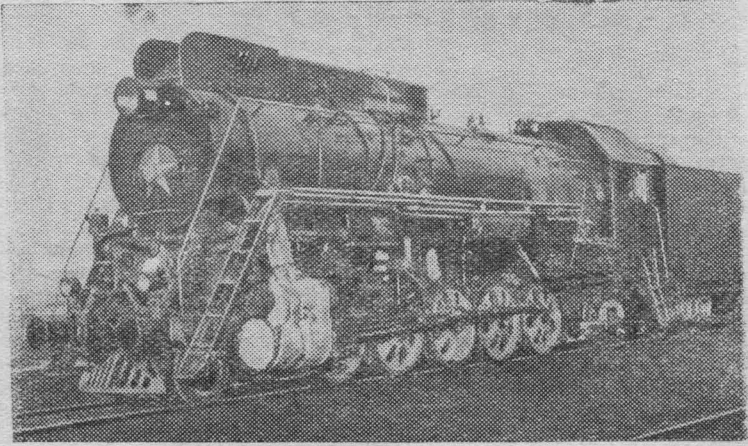
Ворошиловградский паровозостроительный завод имени Октябрьской революции готовится к серийному выпуску мощных паровозов 1-5-1. На снимке: паровоз 1-5-1 перед пробной обкаткой.
