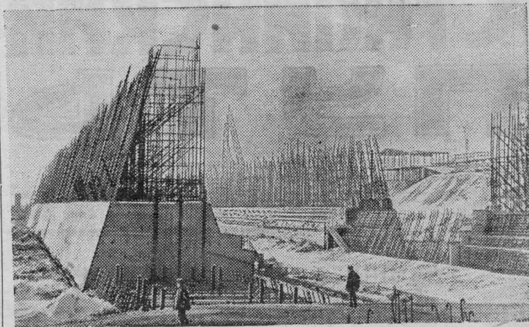
Куйбышевгидрострой. Широким фронтом ведутся работы на первом пусковом объекте гидроузла — нижнем судоходном плёзе. На снимке: общий вид строительства левой камеры нижнего судоходного плёза.
