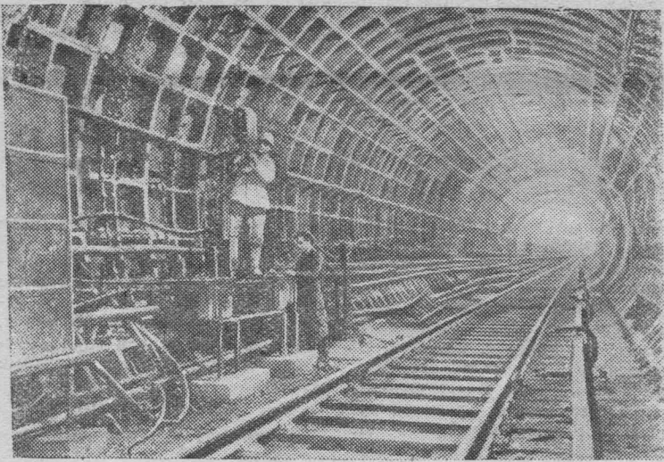
Москва. Строительство Большого кольца метрополитена. На снимке: перегонный туннель между станциями «Краснопресненская» и «Киевская—кольцевая».
