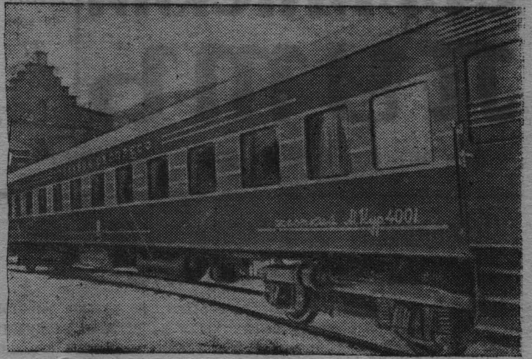
Ленинградский вагоностроительный завод имени Егорова выпустил первый в СССР цельнометаллический пассажирский вагон «Голубой экспресс» на 60 спальных мест. Начат серийный выпуск вагонов этого типа. Первый состав «Голубого экспресса» предназначен для курсирования на линии Москва—Черноморское побережье. На снимке: общий вид первого цельнометаллического вагона.
