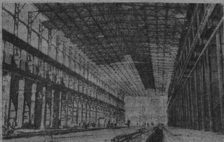
На Брянском паровозостроительном заводе идет строительство главного паровозосборочного пролета площадью 7000 квадратных метров. Одновременно строятся механосборочные цеха. На снимке: общий вид строящегося паровозосборочного пролета.
