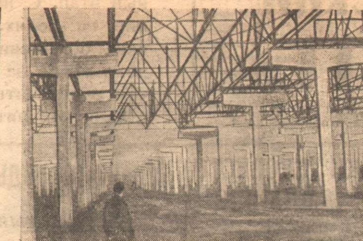
Строительство конвейерного цеха Кутаисского автомобильного завода.
