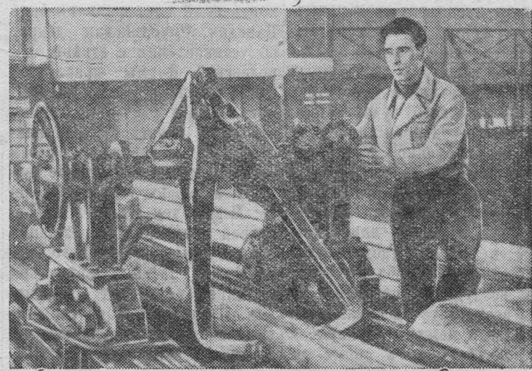
Техник-рационализатор лесопильного завода имени Куйбышева (Сталинград) тов. А. М. Егоров, сконструировавший портативную комлевую тележку для подачи бревен к лесопильной раме. Годовая экономия от одной тележки составляет 26 тысяч рублей. Фото А. Маклецова
