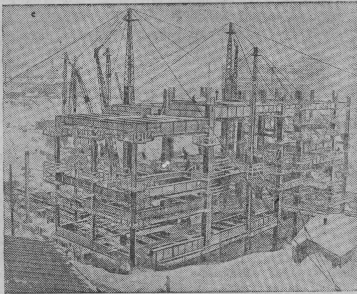
Первые стальные конструкции металлического каркаса нижней части здания Дворца Советов.
