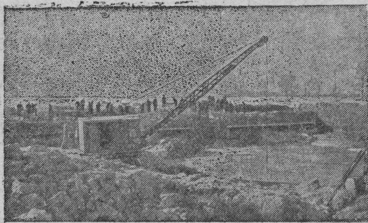
В Западных областях Белоруссии идет строительство Днепро-Бугского канала протяжением в 202 километра. Канал соединит судосходную реку Буг с Днестром и Черным морем. Строительство канала предполагается закончить в апреле текущего года. На снимке: На строительстве 10-го гидроузла Днепро-Бугского канала
