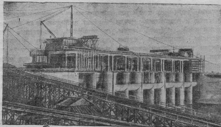
На строительстве Рыбинского гидроузла. НА СНИМKE: общий вид железобетонной плотины № 2.
