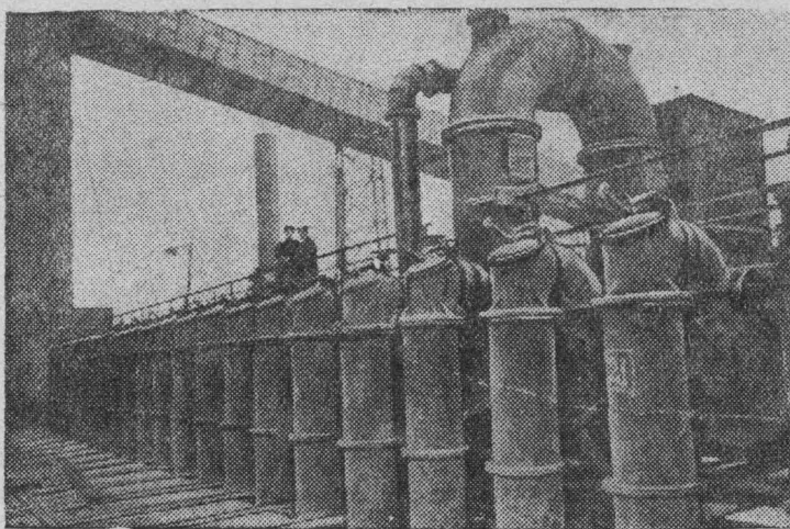
Ново-Тагильский металлургический завод (Свердловская область) в текущем квартале получит от Коксохимзавода кокс и газ. НА СНИМКЕ: Стойки коксовых печей батареи № 2.
