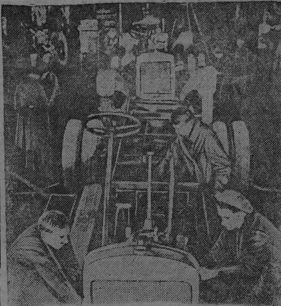
Главный конвейер Харьковского тракторного завода.
