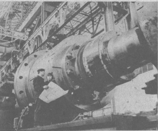
На снимке: обработка вала ротора гидрогенератора мощностью 240 тысяч киловатт.
