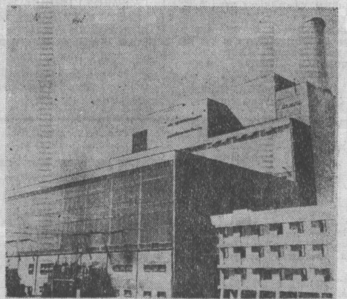
ЮГОСЛАВИЯ. В городе Обреновац при техническом содействии Советского Союза и Чехословакии сооружается тепловая электростанция. СССР поставляет для нее котлы, а СССР — турбины и генераторы. Первый агрегат уже пущен в строй. Закачивается монтаж второго агрегата. После завершения всех работ электростанция «Обреновац» будет одной из самых крупных теплоэлектростанций в Югославии. Ее мощность составит 1600 тысяч киловатт.
