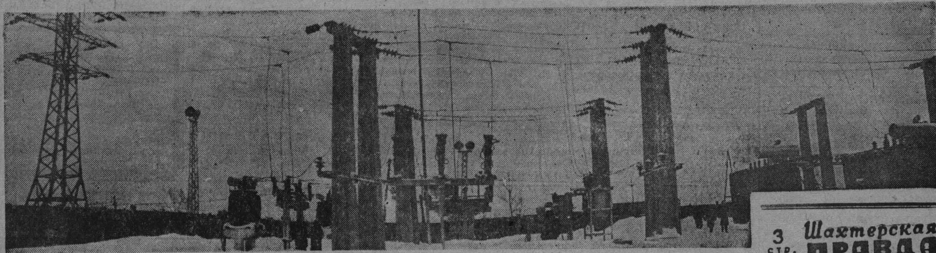
Эта электроподстанция № 31 сетевого района мощностью 15 тысяч киловольтампер питает энергией почти все предприятия и шахты, расположенные в районе Ясной Поляны.
