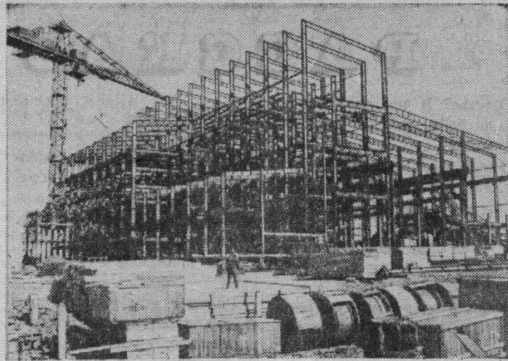
Металлический силуэт строящегося в городе Мирном горнообогатительного комбината виден издали. Для него подобрали прочную скальную площадку за чертой города. Стройка идет полным ходом. Величаво разворачиваются стрелы подъемных кранов, доставляя на верхние этажи металлические балки и перекладины. Это будет самая мощная в нашей стране алмазная фабрика, применяющая передовую отечественную технологию. Когда строительство нового предприятия закончится, кимберлитовая трубка «Мир» даст значительно больше сверкающих кристаллов, так необходимых всем отраслям отечественной промышленности.
