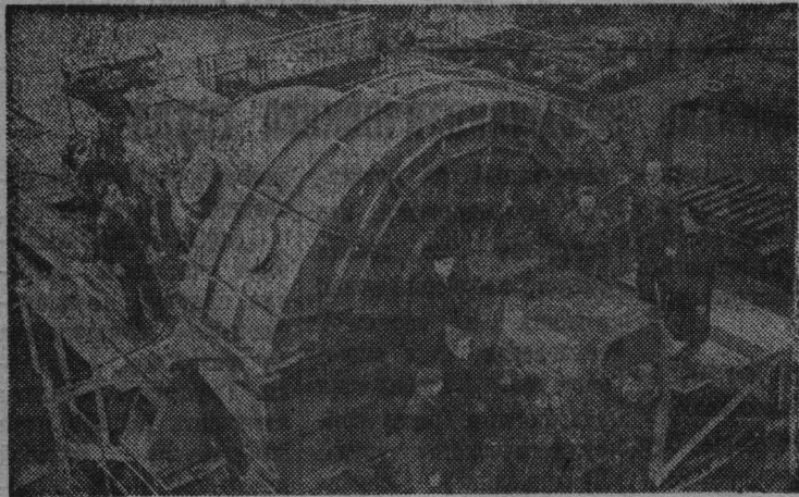
ЛЕНИНГРАД. На Металлическом заводе завершено изготовление крупнейшей в стране газотурбинной установки мощностью 25 тысяч киловатт.
