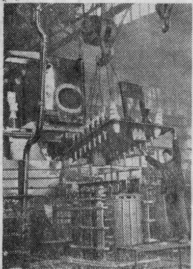
На снимке: сборка трансформатора.
