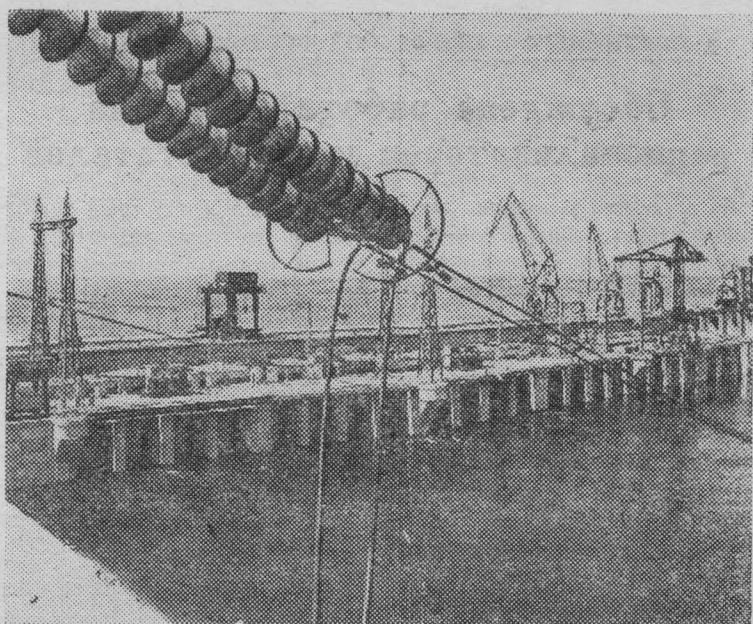
Украинская ССР. Строительство Кременчугской ГЭС подходит к концу. Ныне действующие 7 агрегатов этой мощной электростанции на Днепре выработали более 200 миллионов киловатт-часов электроэнергии. Остальные 5 агрегатов строители решили сдать в эксплуатацию к 43-й годовщине Великого Октября.
