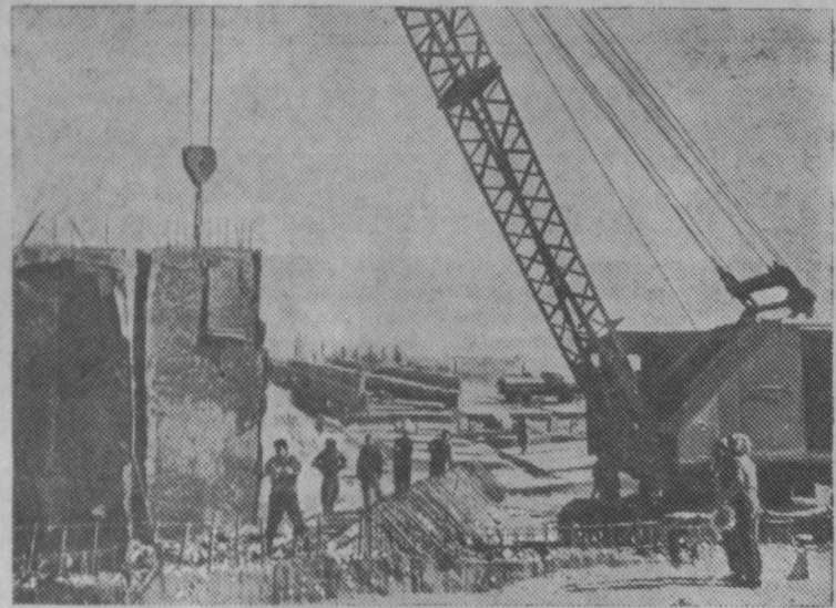
Туркменская ССР. Между Мургабом и Тедженем, там, где ведется строительство второй очереди Кара-Кумского канала, раскинулась огромная строительная площадка Хауз-Ханского водохранилища. Сейчас завершается строительство сопрягающих сооружений в местах ввода и вывода из него искусственной реки.
